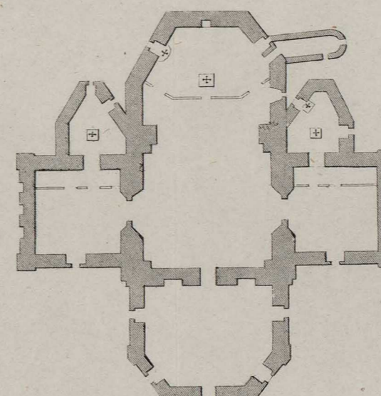
Планъ купола Собора на Софійской площади въ Кіевѣ, сооруженнаго Д. М. Младшимъ.
